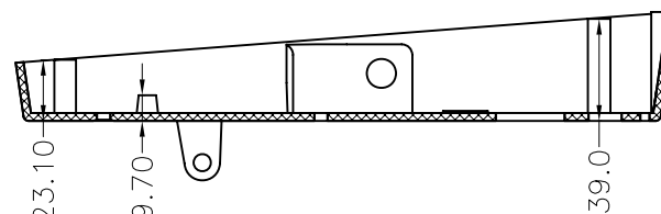
剖面 A-A
