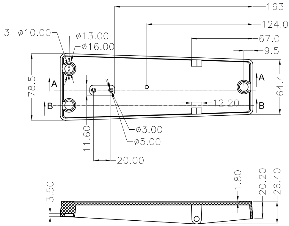
剖面 A-A
