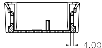
剖面 B-B
