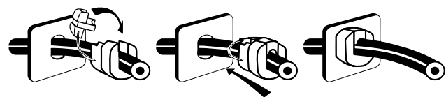
Instrução de montagem do prensa cabos
